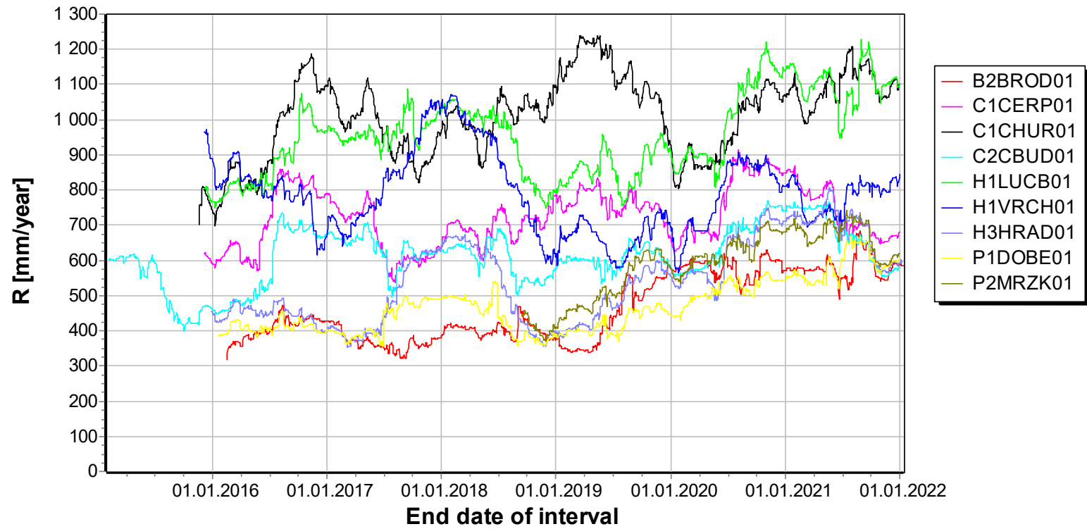
Obr. 2. Klouzavý roční (365-tidenní) úhrn srážek na vybraných stanicích za dobu vyhodnocení dat. Running annual (365-day) sum of precipitations at selected stations during the data evaluation.
