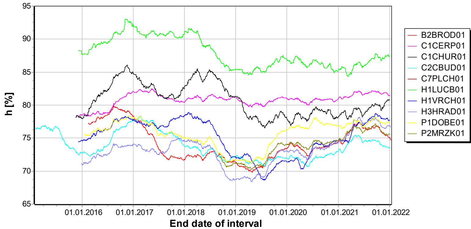
Obr. 3. Klouzavý roční (365-tidenní) průměr relativní vlhkosti vzduchu na vybraných stanicích za dobu vyhodnocení dat. Running annual (365-day) average of air humidity at selected stations during the data evaluation.
